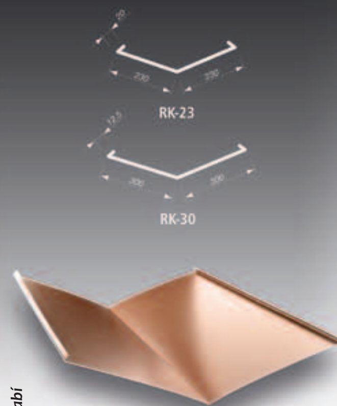
Hřeben pro plechovou střešní krytinu Venecia
